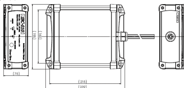
概略寸法図
