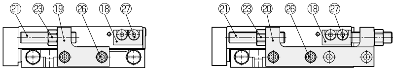
金属ストッパ 押出側ストローク調整タイプ 金属ストッパ 両側ストローク調整タイプ
