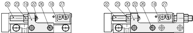
ラバーストッパ 押出側ストローク調整タイプ ラバーストッパ 両側ストローク調整タイプ
