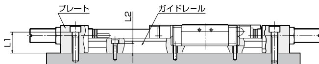
プレート部 取付ボルト
