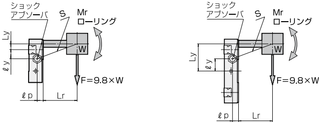
ローリング (SD、WGガイド)
