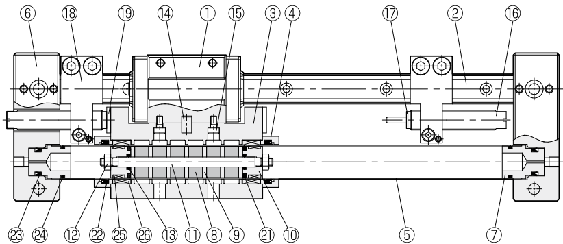
ストップパ方式: QA (エンドプレート式)
