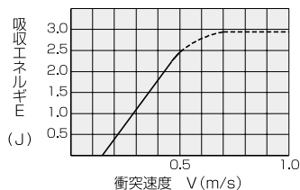
吸収エネルギー グラフ
