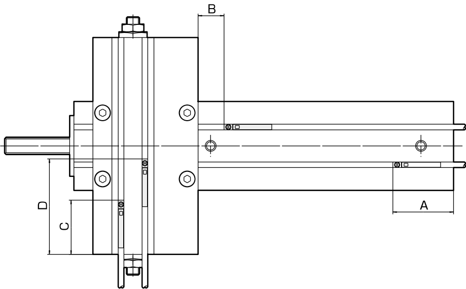
RB1、2 RC1スイッチ
