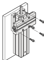
ブラケット金具取付 （貫通穴）
