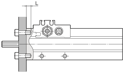
前面からの取付 (ボディタップ)
