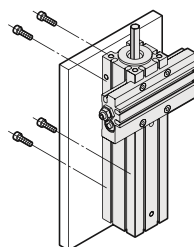
底面からの取付 （ボディタップ）
