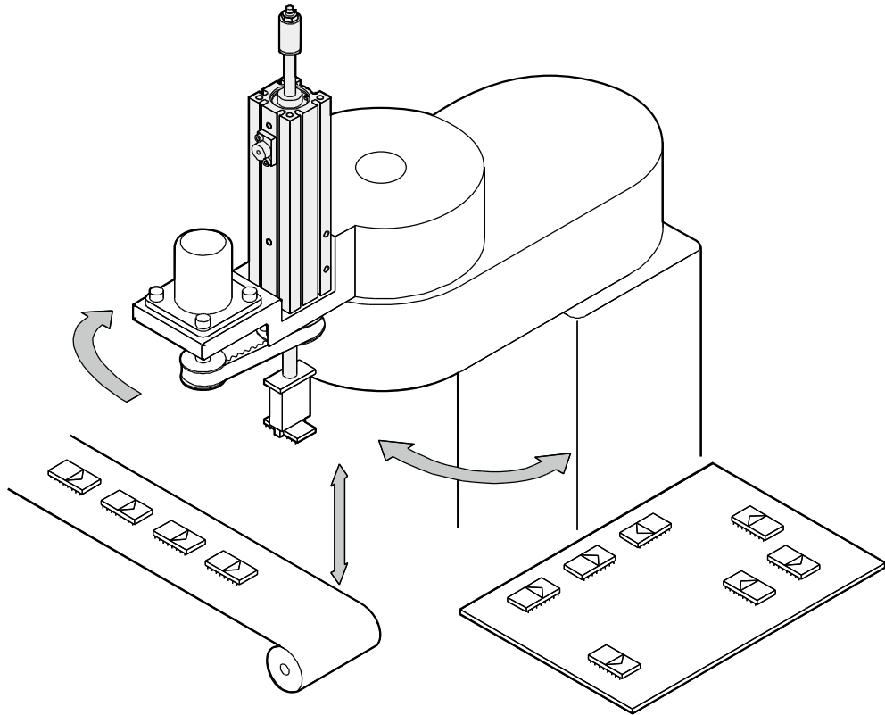
実装ロボット
