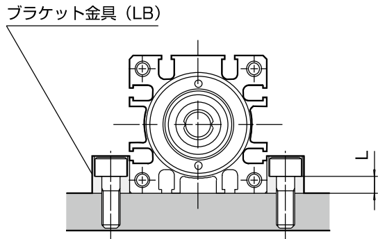
ブラケット金具 (LB) 取付
