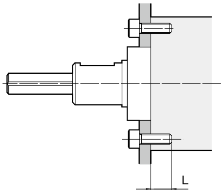
前面からの取付（ボディトップ）
