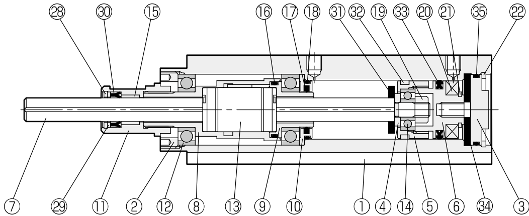
ストローク調整機構付
