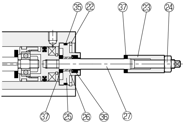
ストローク調整機構付
