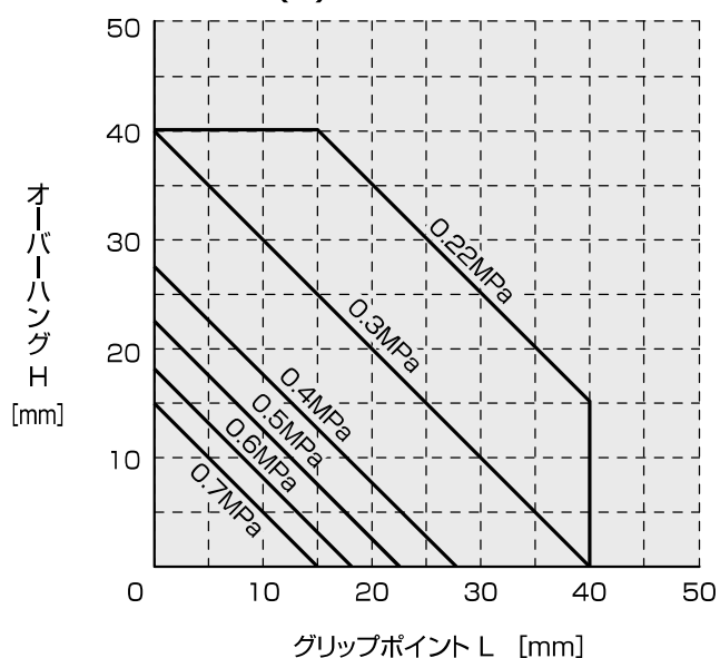
NEOK(F)-8C
