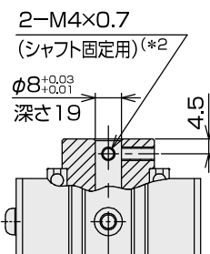
2:穴タイプ
