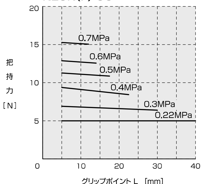
NEOK(F)-8C
